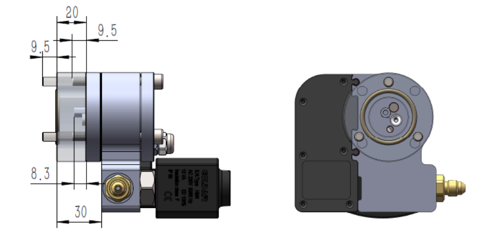
OUT680R-1 带GOA20F 法兰加高块与短款喷油管
