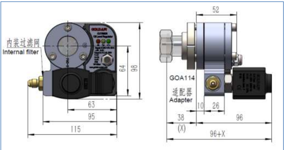
图 1：外形尺寸 Figure 1: Dimensions
