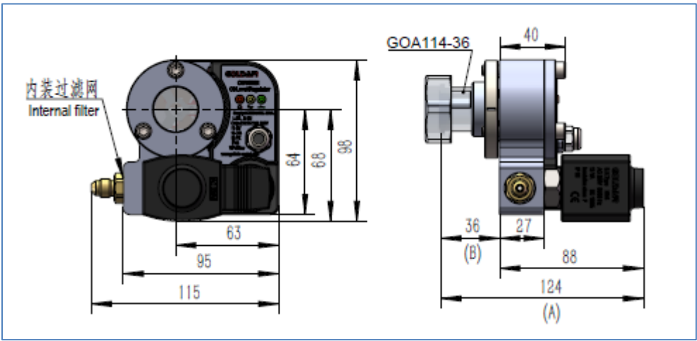
图 1：外形尺寸 Figure 1: Dimensions
